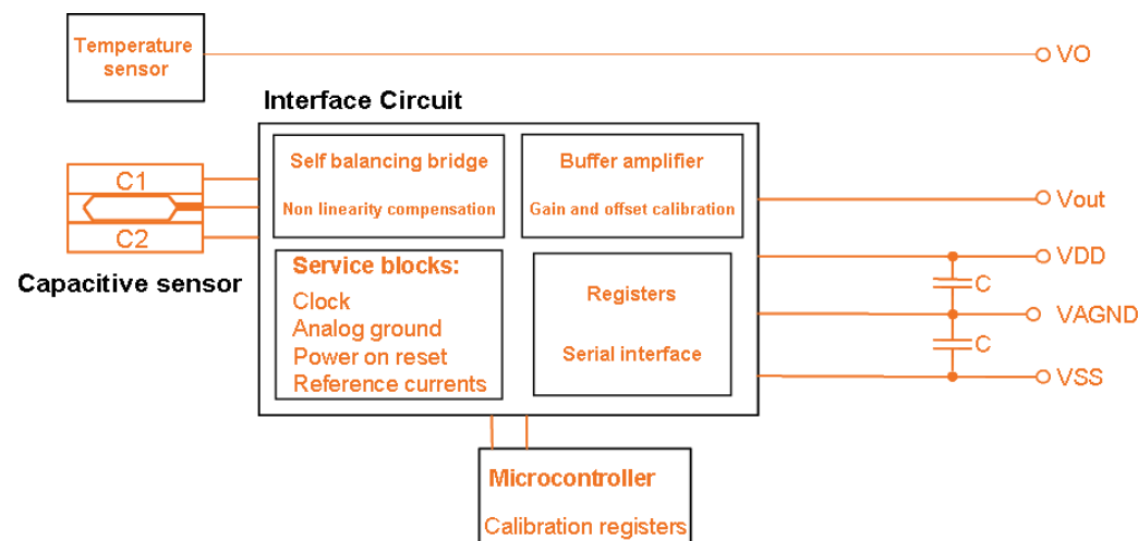
Fig. 4 : Block diagram
